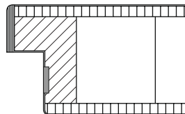
Starkfurnier Kante mit Furnierkante im Falz, Brandschutzquellstreifen sichtbar
